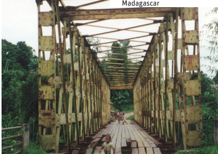
Rénovation du pont PK48 Madagascar
