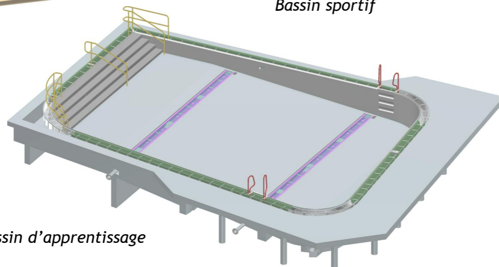
Bassin sportif
