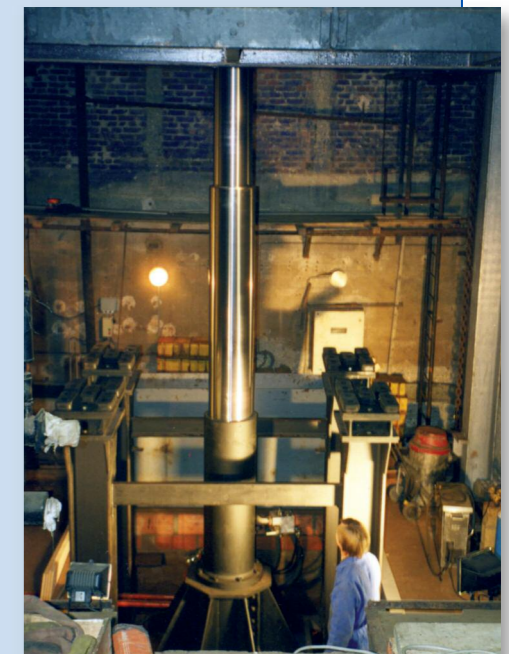
Machinerie d'élévation de la piscine (vérin sorti totalement)
