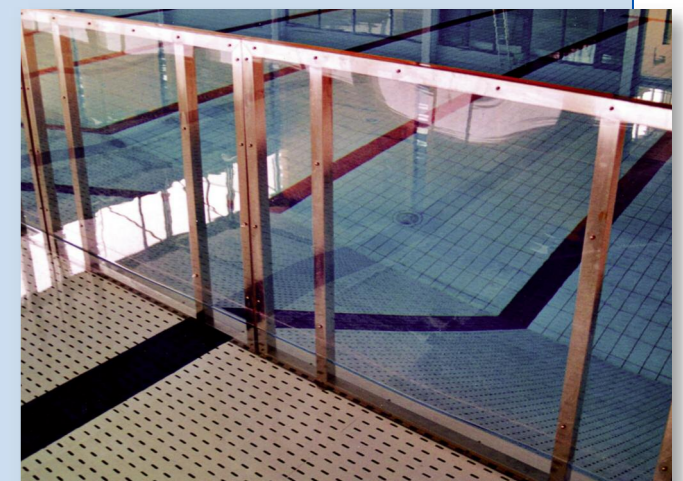
Détail garde-corps et plancher
