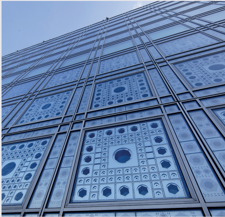
Automatisation des moucharabihs de l'Institut du Monde Arabe
