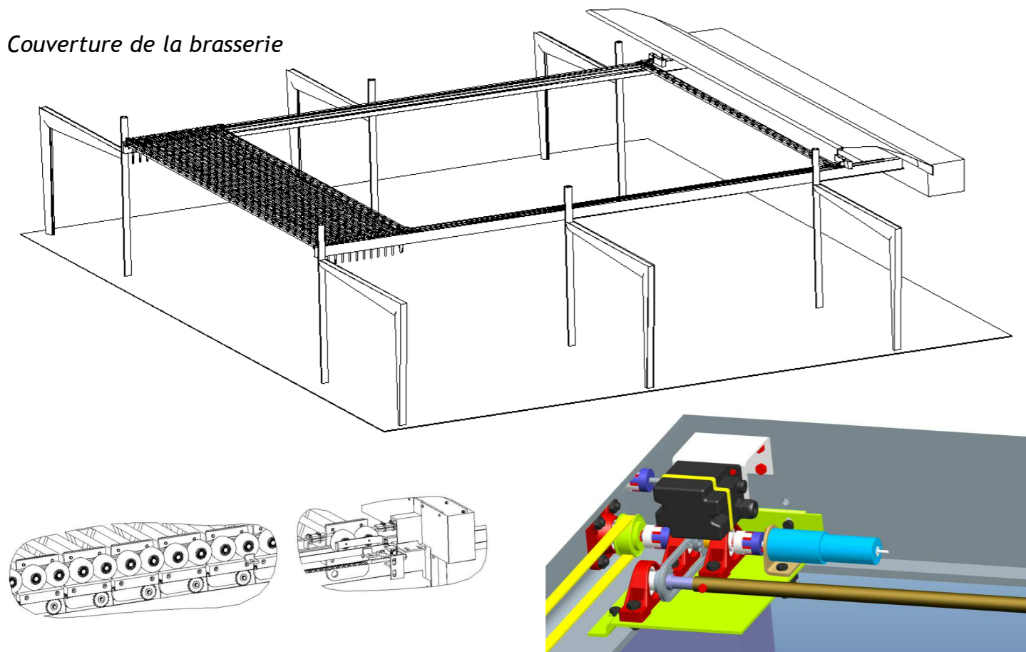
Motorisation de la couverture de la brasserie
