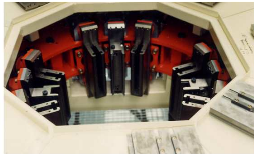
presse de frettage
